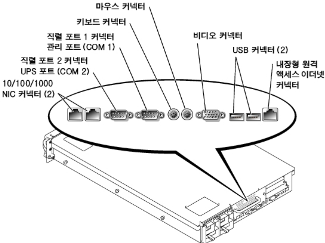
그림 B-1. 후면 패널 I/O 포트 및 커넥터
