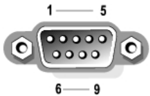
그림 B-3. 직렬 포트 핀 번호
