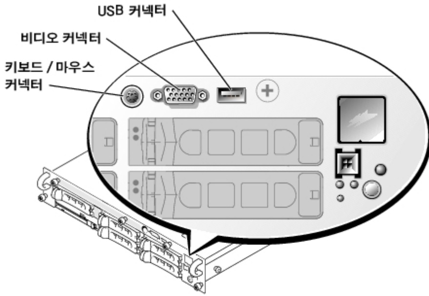
그림 B-2. 전면 패널 I/O 포트 및 커넥터
