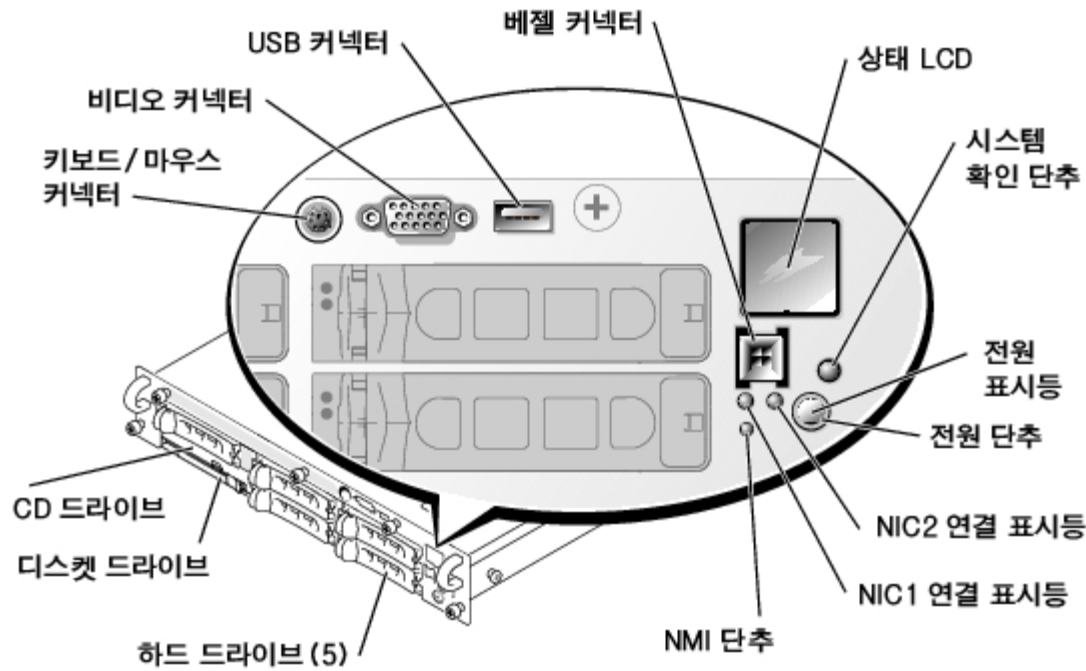
그림 1-2. 전면 패널 구조
